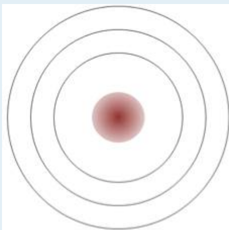
Beryllium (3)
