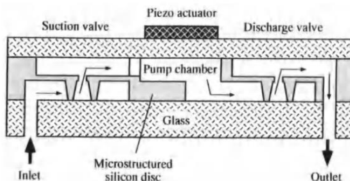
Fig.6. Micro membrane pump
