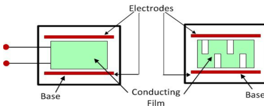
Fig. 28. Hygrometer
