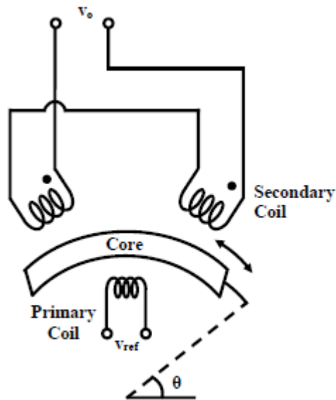
Fig.12. RVDT
