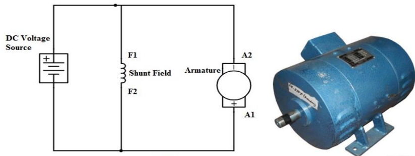
Fig.6. Shunt motor
