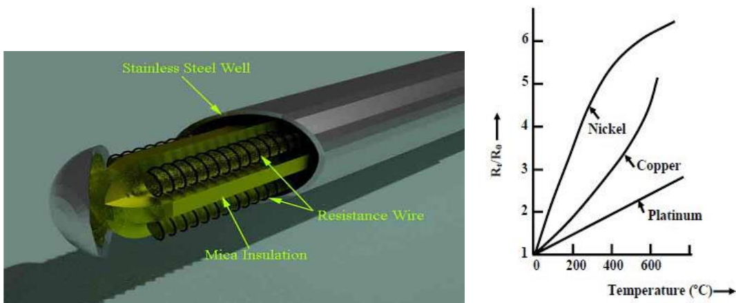
Fig. 21. a) RTD b) waveform
