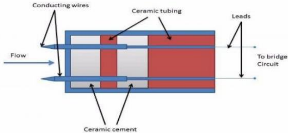
Fig. 24. Hot Wire Anemometer
