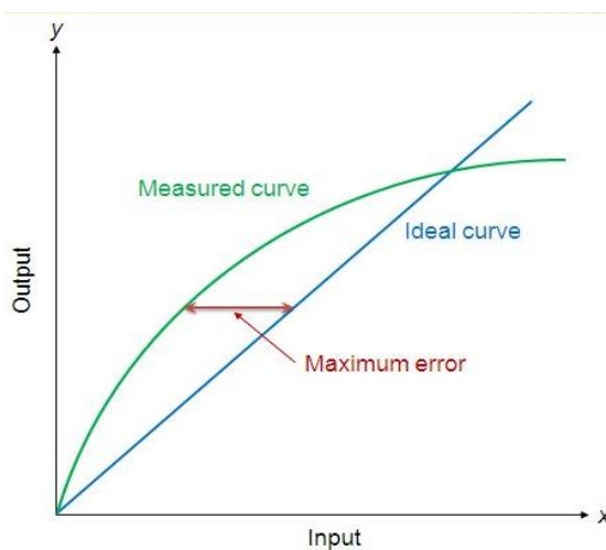
Fig. 3. Non linearity
