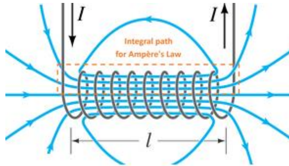
Fig.4. Solenoid
